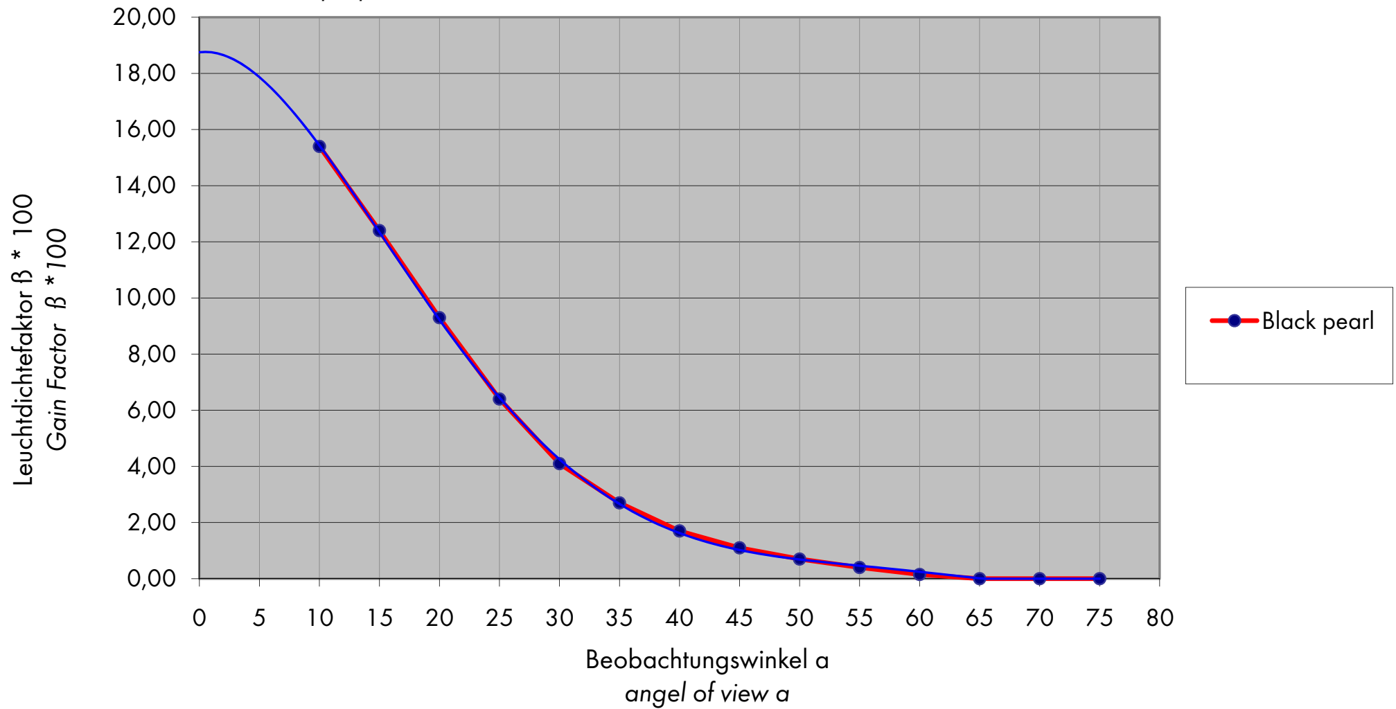
Projektionsfolie BLACK PEARL - Reflexion nach DIN 19045-4 projecion screen BLACK PEARL - reflexion acc. to DIN 19045-4
