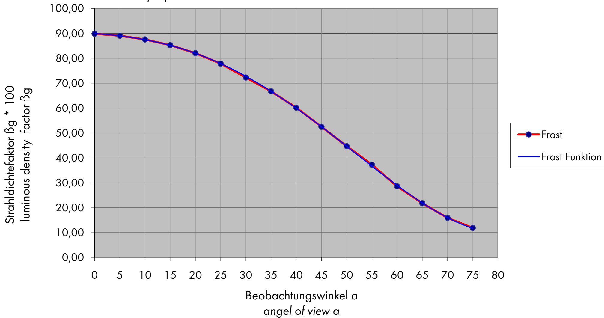
Projektionsfolie FROST - Transmission nach DIN 5036-3 projeccion screen FROST - transmission acc. to DIN 5036-3
