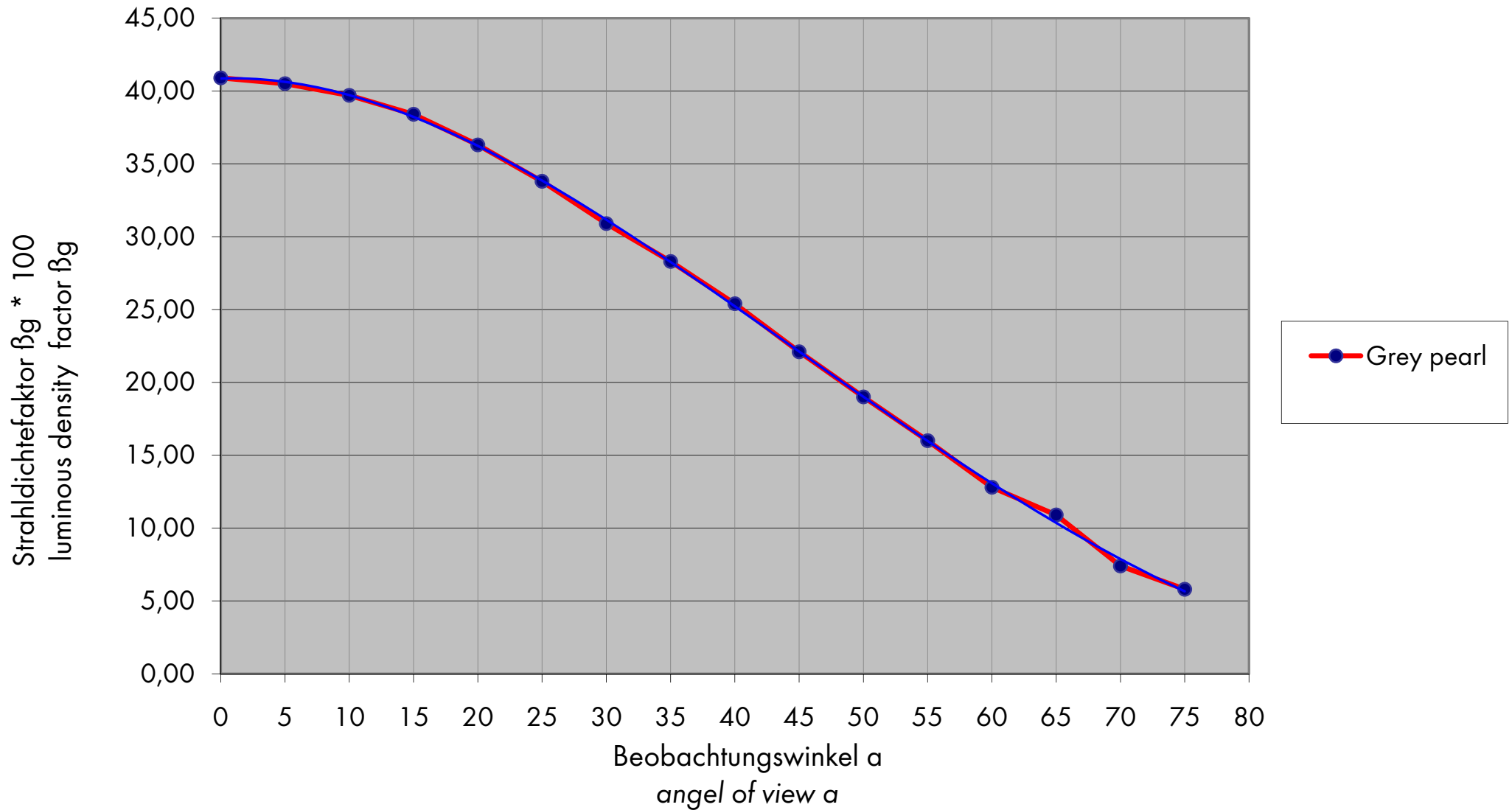
Projektionsfolie GREY PEARL - Transmission nach DIN 5036-3 projecion screen GREY PEARL - transmission acc. to DIN 5036-3
