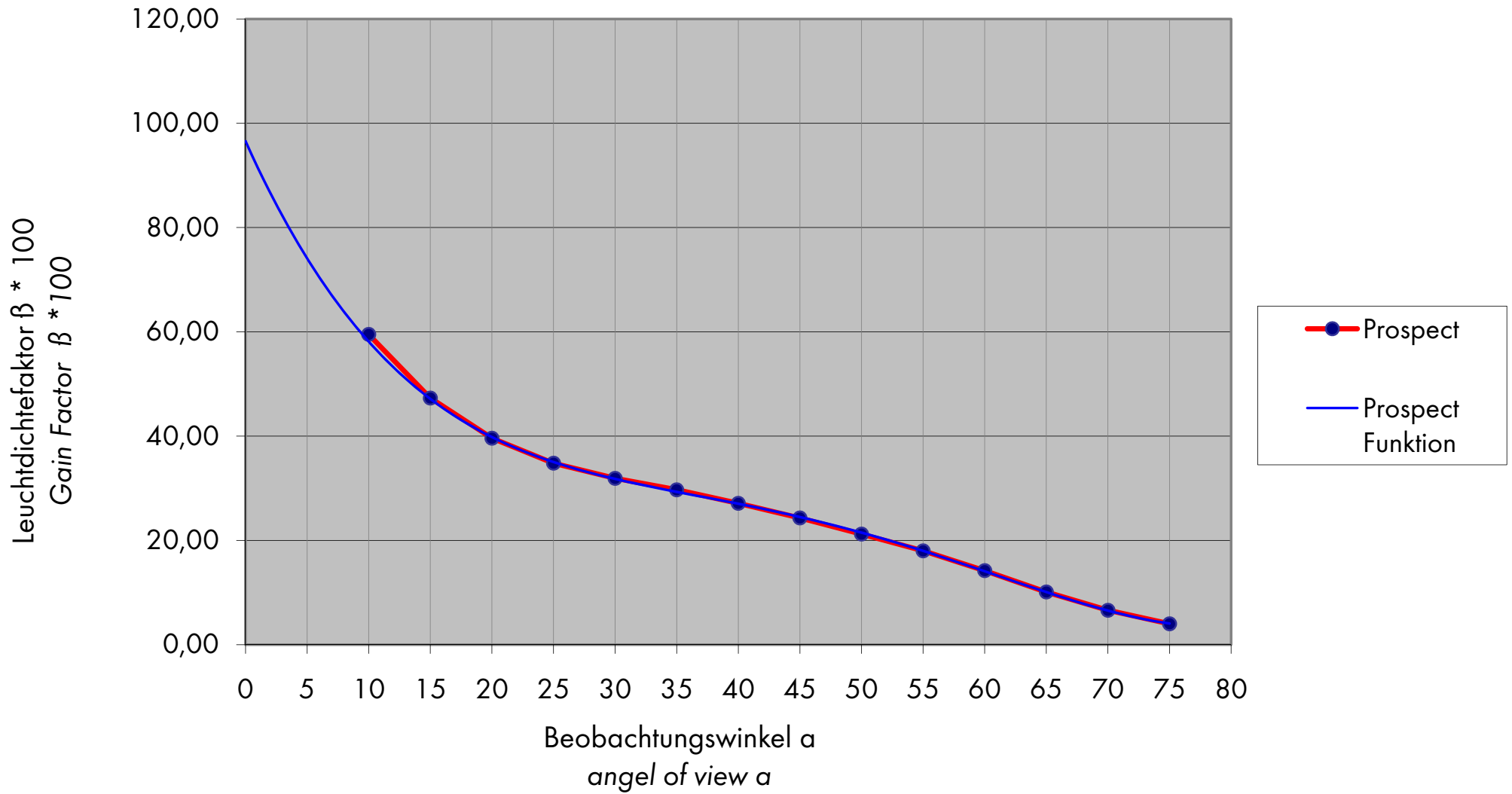
Projektionsfolie PROSPECT- Reflexion nach DIN 19045-4 projection screen PROSPECT - reflexion acc. to DIN 19045-4
