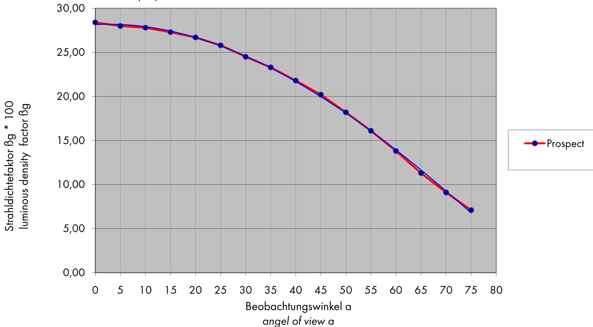
Projektionsfolie PROSPECT - Transmission nach DIN 5036-3 projecion screen PROSPECT - transmission acc. to DIN 5036-3
