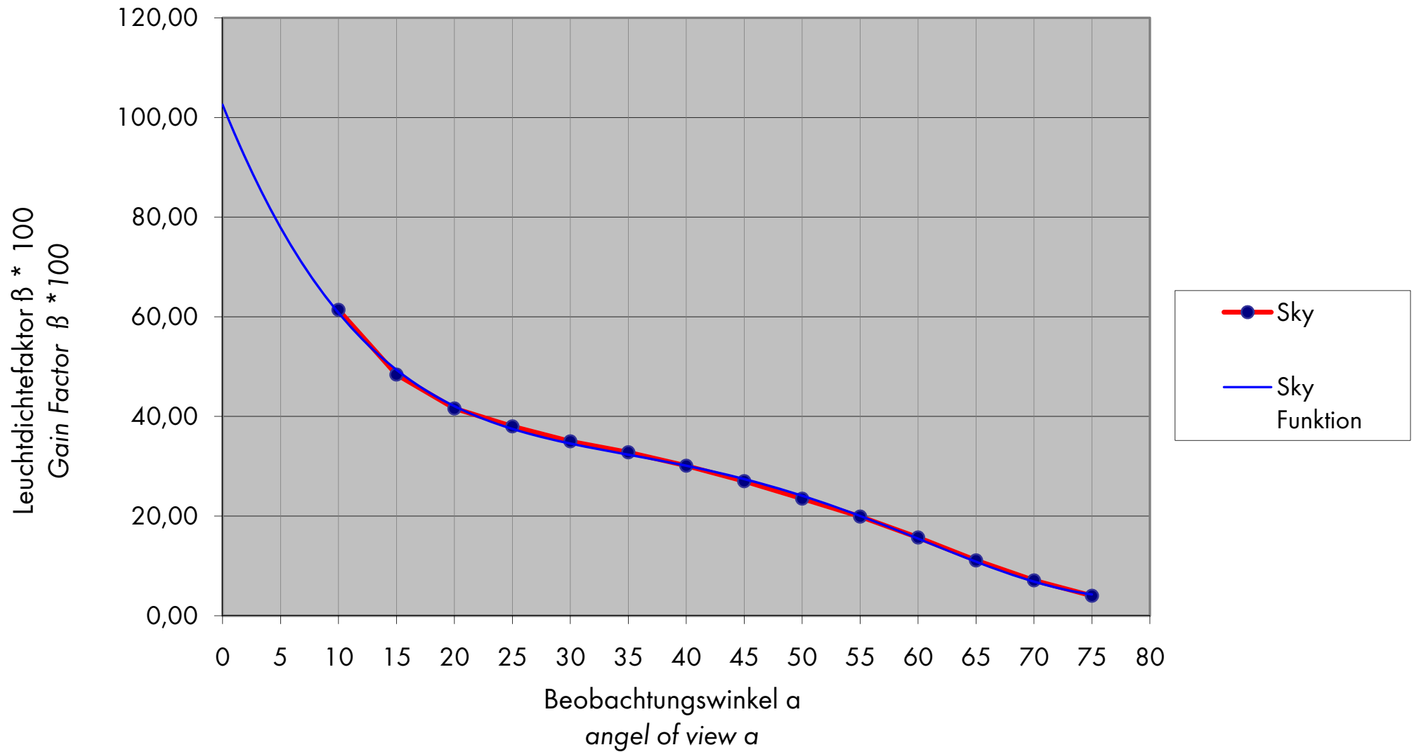
Projektionsfolie SKY - Reflexion nach DIN 19045-4 projection screen SKY - reflexion acc. to DIN 19045-4
