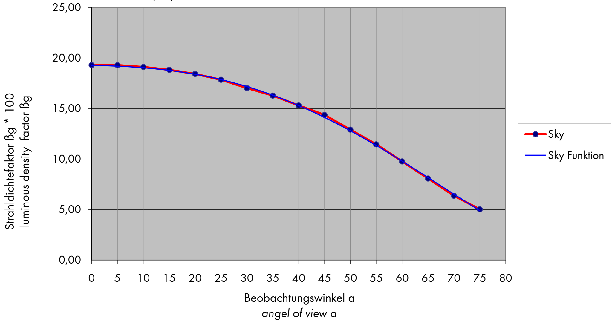
Projektionsfolie SKY - Transmission nach DIN 5036-3 projeccion screen SKY - transmission acc. to DIN 5036-3
